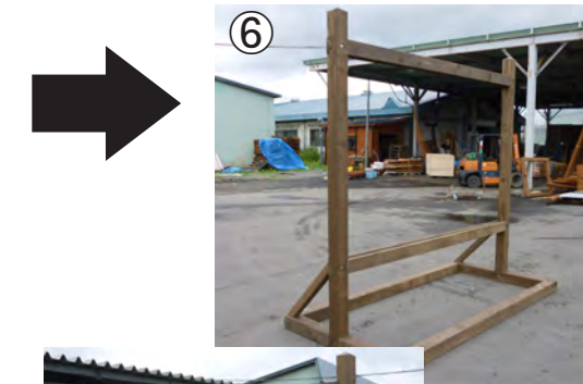
【下台（横柱，縦柱）】 × 各2本
